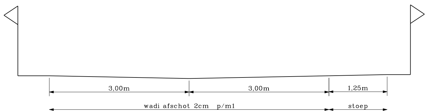
Dwarsprofiel A - A Schaal 1:50
